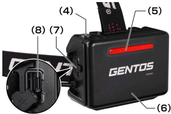
(4)後部認識灯スイッチ (5)後部認識灯 / チャージングインジケータ (6) 電池カバー (7) USB Type-Cポートカバー (8) USB Type-Cポート
