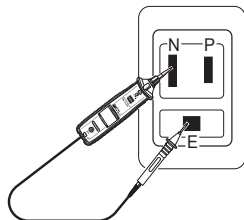
図8-4 コンセントの接地抵抗を測定
