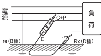
図8-3 負荷の接地抵抗を測定
