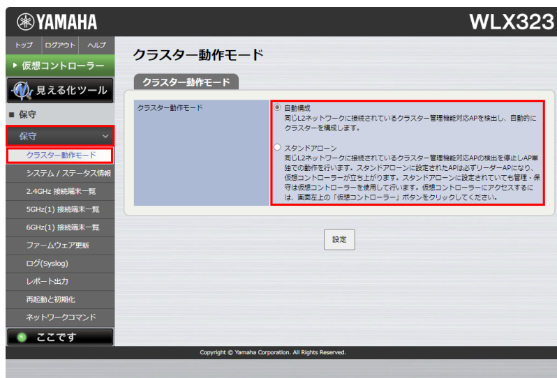
無線APのWeb GUI [トップ] - [保守] - [クラスター動作モード]
