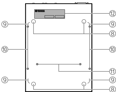
【SWX2210P-10G】
