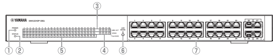
SWX2210P-18G
