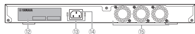
SWX2210P-18G
