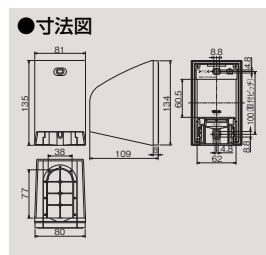
引込カバー(防雨形) DC7301(T) ¥1,300○ ●φ20(5) ●防雨形(IPX3) ※スイッチボックス取り付け不可 ●ブラウン色
