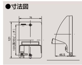
入線カバー(防雨形) DC7022(T) ¥700○ ●φ50(5) ●防雨形(IPX3) ●コード押え付 ●JIS規格1コ用露出ボックス対応 ●ブラウン色
