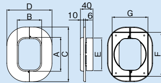
寸法図
