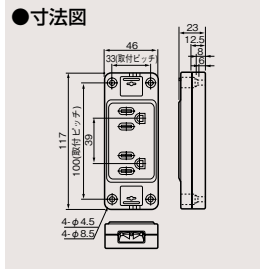
SL角形アース付ダブルコンセント DC1262E ¥680○ ●15A-125V AC ●●100(20)
