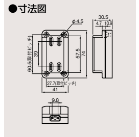
SL角形ダブルコンセント DC1222N ¥460○ ●15A-125V AC ●●100(20)
