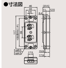
SL角形抜止接地ダブルコンセント DC1292E ¥970○ ●15A-125V AC ●●100(20)
