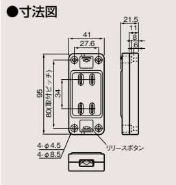
SL角形ダブルコンセント DC1262 ¥460○ ●15A-125V AC ●●200(20)
