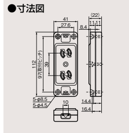
SL角形抜止ダブルコンセント DC1292 ¥780○ ●15A-125V AC ●●100(20)
