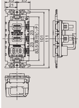
●寸法図
