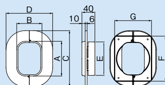
寸法図
