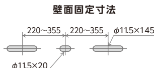
壁面固定寸法
