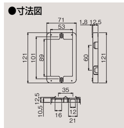
WIDE-i プレート継枠(1連用) WDG7591(CW) ¥360 ○ ●φ50(5) ●ウォームベージュ色
