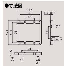
WIDE-i プレート継枠(2連用) WDG7592(WW) ¥490 ○ ●φ20(-) ●ニューホワイト色
