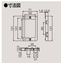
WIDE-i プレート継枠(1連用) WDG7591(WW) ¥360 ○ ●φ50(5) ●ニューホワイト色
