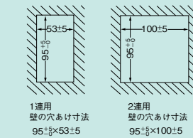
パネル押え金具(7~18mm壁用) NDG4332 ￥85 ○ ●7~18mm用 ●φ200(20) ●付属ねじ2本(M4×20)
