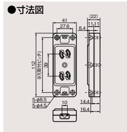
仮設用 SL角形抜止ダブルコンセント DC1292 ¥780○ ●15A-125V AC ●●100(20)
