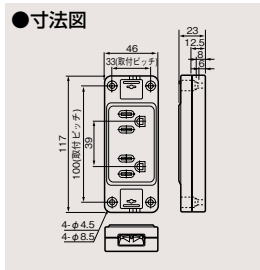
仮設用 SL角形アース付ダブルコンセント DC1262E ¥680○ ●15A-125V AC ●●100(20)
