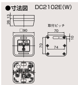
2P接地付30A露出コンセント DC2102E(W) ¥2,450○ ●30A-250V AC ●●50(1) (送りなし) ●圧着端子3個付属
