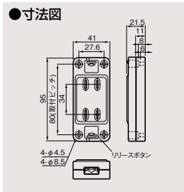
仮設用 SL角形ダブルコンセント DC1262 ¥460○ ●15A-125V AC ●●200(20)
