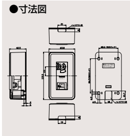
露出アースターミナル付 抜止接地コンセント DC1381E(WW) ¥1,340○ ●15A-125V AC ●●50(5)
