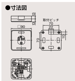
小型接地2P30A露出コンセント DC2252E(W) ¥2,050○ ●30A-250V AC ●●20(10) (送りなし) ●圧着端子3個付属
