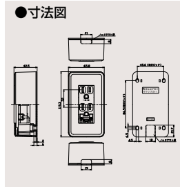
露出アースターミナル付 接地ダブルコンセント DC1182E(WW) ¥1,280○ ●15A-125V AC ●●50(5)
