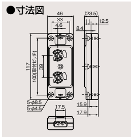
仮設用 SL角形抜止接地ダブルコンセント DC1292E ¥970○ ●15A-125V AC ●●100(20)
