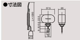
キャノピースイッチ DS2611C ¥420 ○ ●3A-300V AC ●●100(10) ●ひも全長1000mm (出荷時にひもはスイッチに結ばれていません。)
