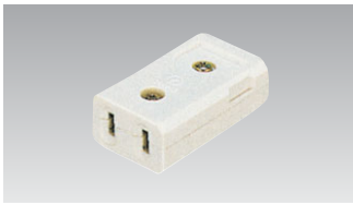
コードコネクタボディ DH7172 ¥150 ○ ●15A-125V AC ●●200(20) ●ホワイト色 適合コード：平形コード0.75mm 2 ～2mm 2
