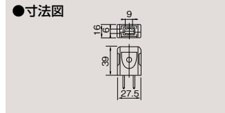
平形キャップ DH1072 ¥120 ○ ●15A-125V AC ●●400(20) 適合コード：平形コード0.75mm 2 ～2mm 2
