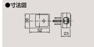
横出しアース付キャップ DH1182E ¥470 ○ ●15A-125V AC ●●100(10) 適合コード：ビニルキャブタイヤ丸形コード3心 VCTF 0.75mm 2 /1.25mm 2 /2mm 2 ゴム絶縁キャブタイヤ丸形コード CTF 0.75mm 2 /1.25mm 2 /2mm 2
