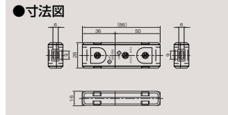
コードコネクタ DH7072 ¥270 ○ ●15A-125V AC ●●200(20) ●ホワイト色 適合コード：平形コード0.75mm 2 ～2mm 2
