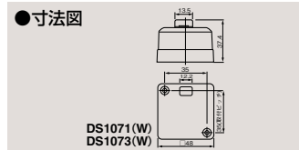
角形タンブラスイッチ(3路) DS1073(W) ¥500 ○ ●10A-300V AC ●●100(10)
