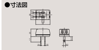
3角タップ DH8143(W) ¥220 ○ ●15A-125V AC ●●100(10) ●ホワイト色 ●3コ用
