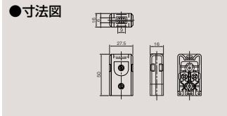
コードコネクタボディ DH7172 ¥150 ○ ●15A-125V AC ●●200(20) ●ホワイト色 適合コード：平形コード0.75mm 2 ～2mm 2
