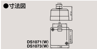
角形タンブラスイッチ(片切) DS1071(W) ¥290 ○ ●10A-300V AC ●●100(10)
