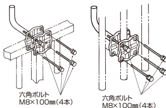
設置例 〈笠木への取付け〉 〈格子への取付け〉
