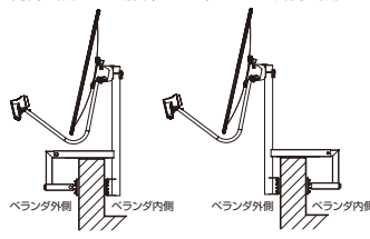
設置例 〈マストを内側に設置した場合〉 〈マストを外側に設置した場合〉
