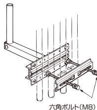
設置例 〈格子への取付け〉
