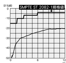
BCP-TKのリターンロス
