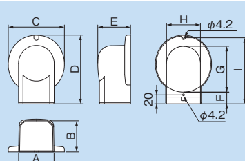
寸法図
