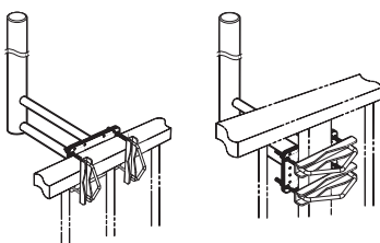
設置例 〈笠木への取付け〉
