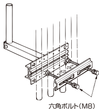
設置例 〈格子への取付け〉
