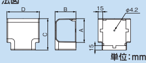
寸法図
