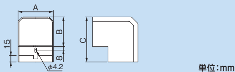
寸法図
