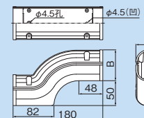
寸法図
