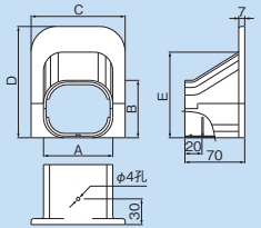
寸法図
