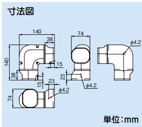
寸法図
