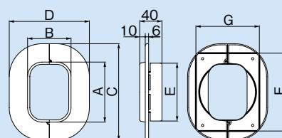
寸法図
