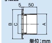
寸法図
