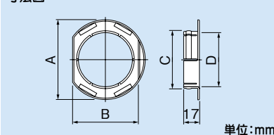
寸法図
