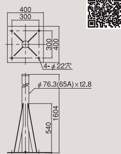
寸法図 (mm)
