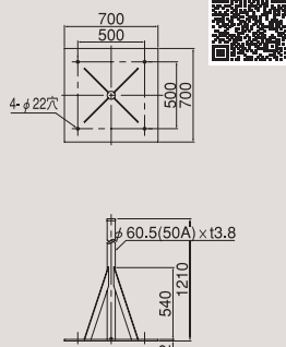
寸法図 (mm)
