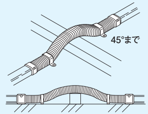
立体曲げ
