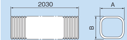
寸法図
