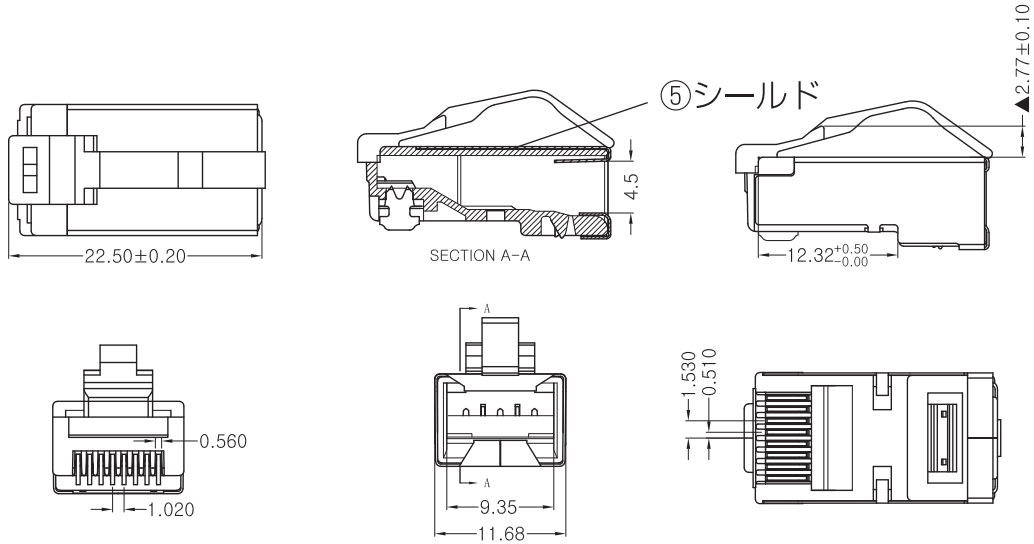
① 本体
