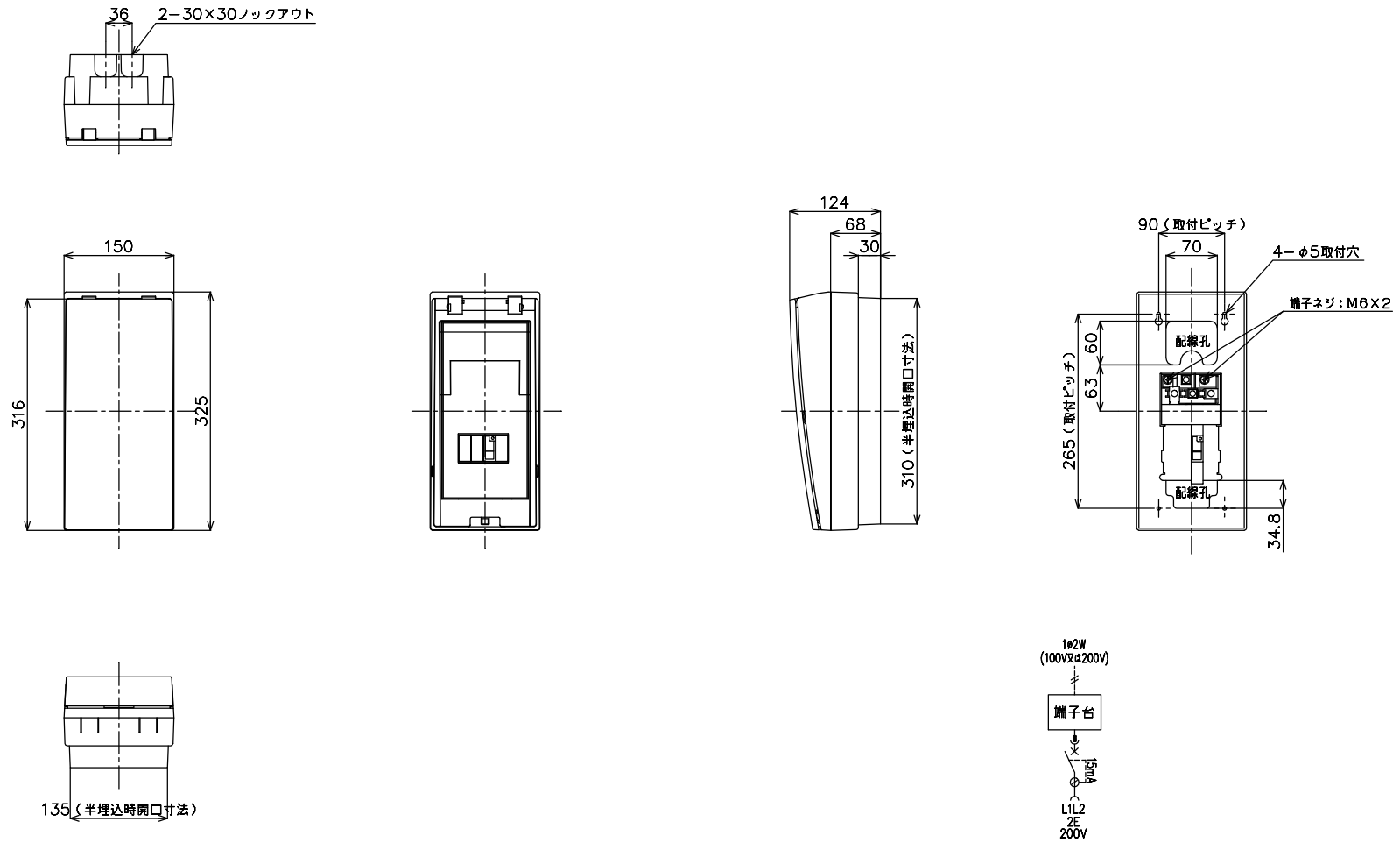
EV/PHEV充電用) 端子台 SHE2P2E20A 15mA (BSHE22022)
