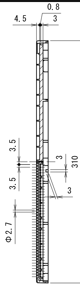
断面 A-A
