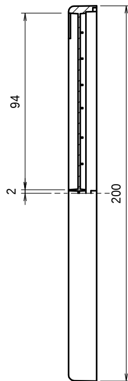
B-B断面図
