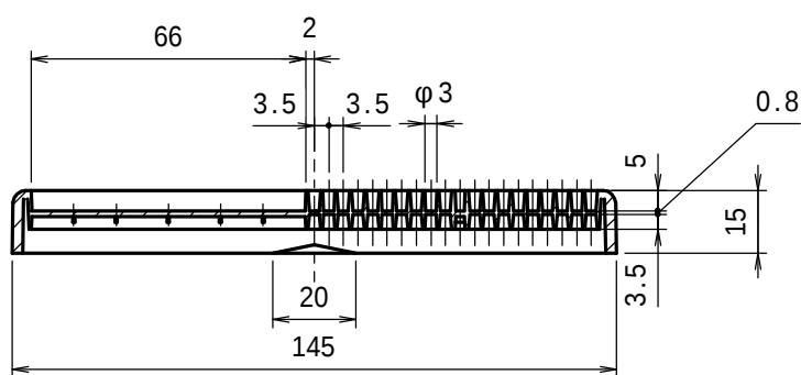
A-A断面図
