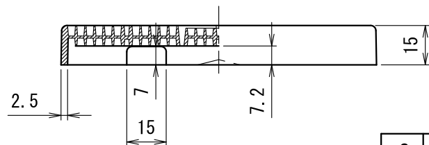
B-B断面図
