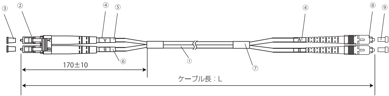
ケーブルの構造
