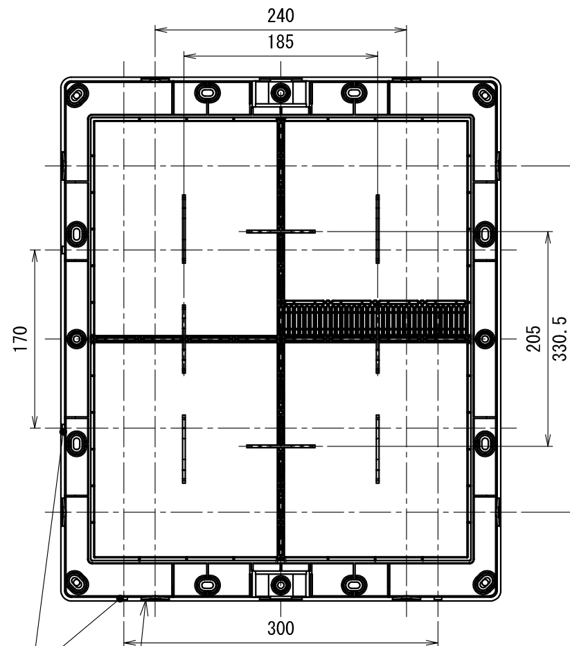
通線ノック8ヶ所
