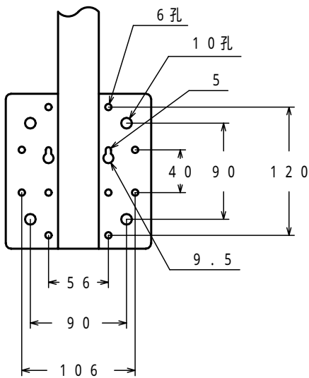
取付孔寸法図
