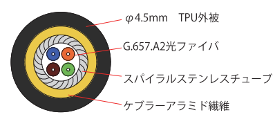
ケーブル断面図
