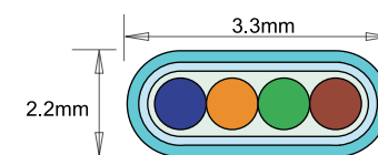
4 芯テープコード 1.青 2.橙 3.緑 4.茶
