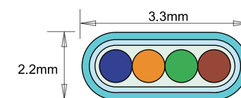
4 芯テープコード 1.青 2.橙 3.緑 4.茶
