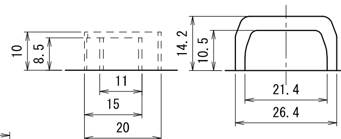
側面ロックアウト B 詳細 (1/1)
