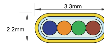
4心テープコード 1.青 2.橙 3.緑 4.茶
