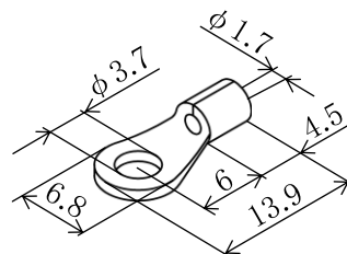
バラ端子 (ニチフ製：R1.25-3.5M)
