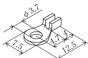
連続端子 (日本圧着端子製：SRA-50T-3.7)
