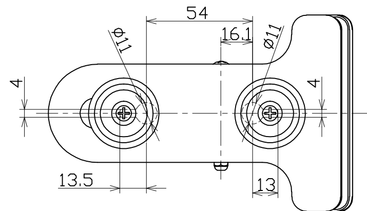
A矢視図
