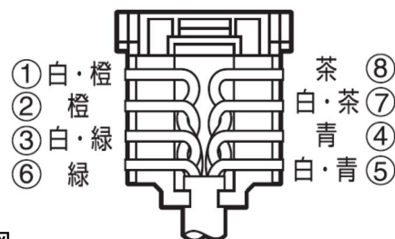
T568B
