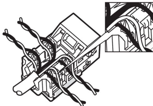
T568A
