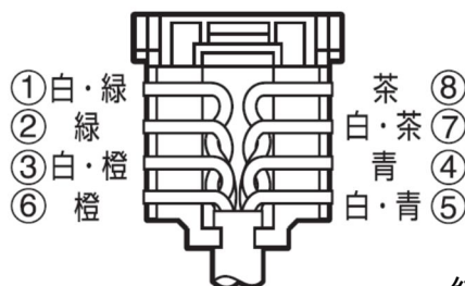
T568A
