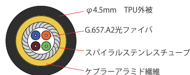
ケーブル断面図
