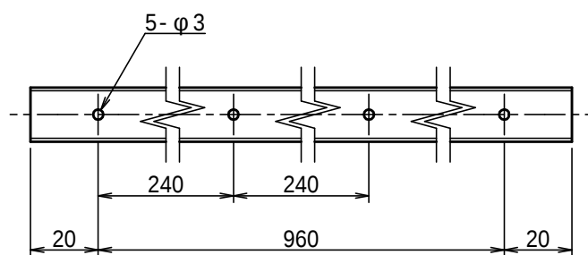
製品裏面釘穴図
