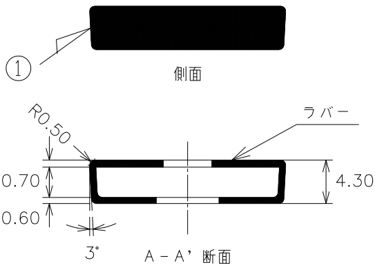
A-A' 断面
