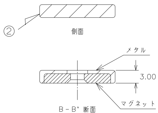
B-B' 断面
