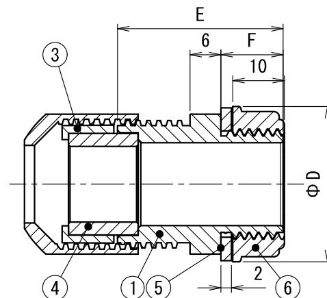
断面 A-A
