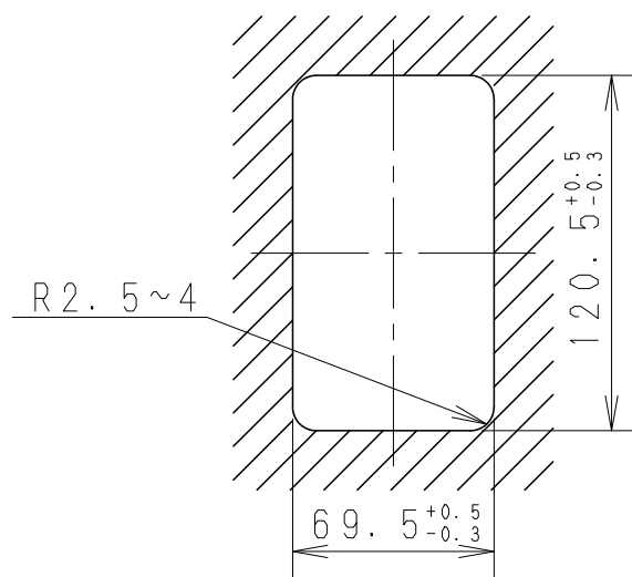
パネルカット寸法図
