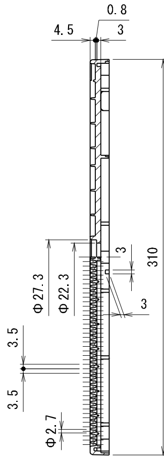
断面 A-A
