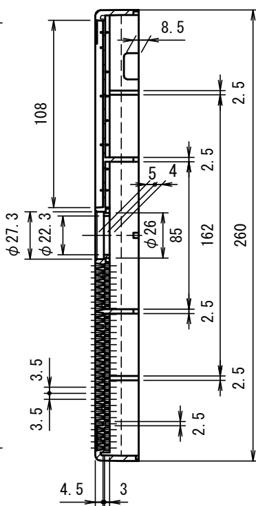
A-A断面図
