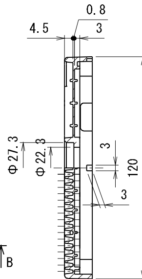
断面 A-A
