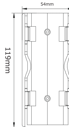
収納専用ホルダー 寸法
