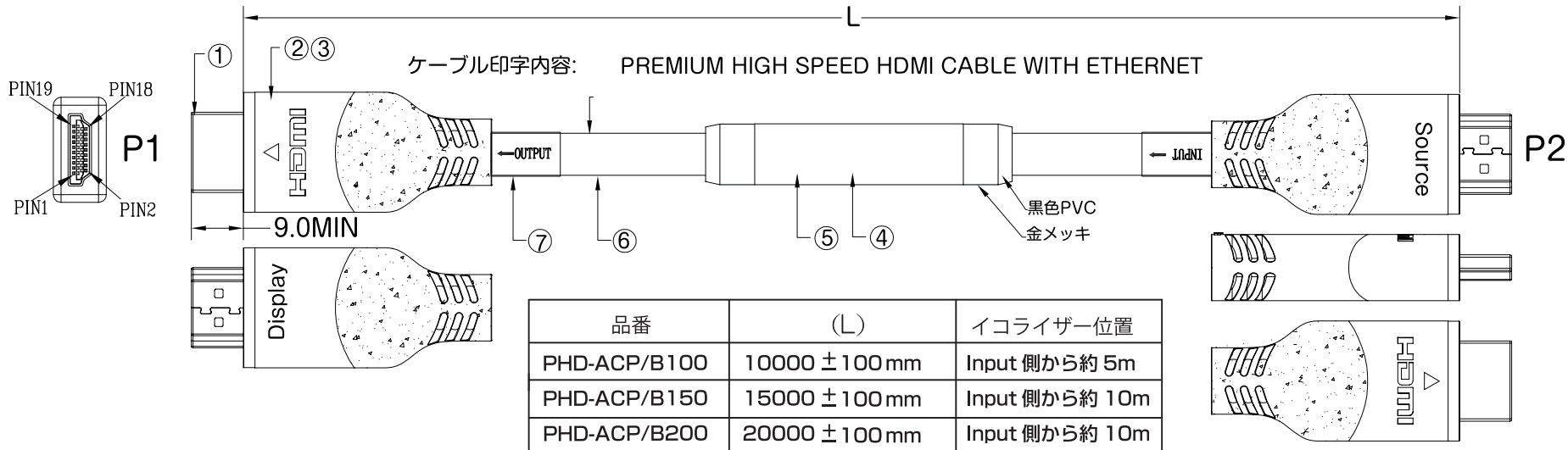
ピンの配列
