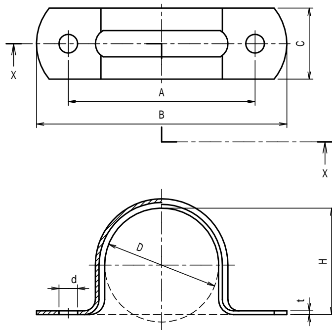
X-X断面図
