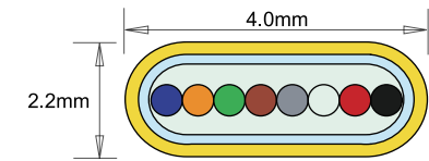
8 芯テープコード 1.青 2.橙 3.緑 4.茶 5.灰 6.白 7.赤 8.黒
